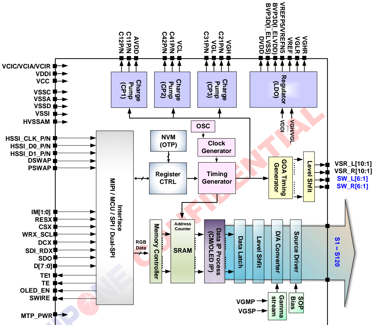
ICNA3306 Block diagram
